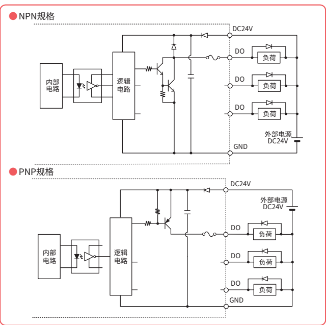
■ 输出信号连接示例
