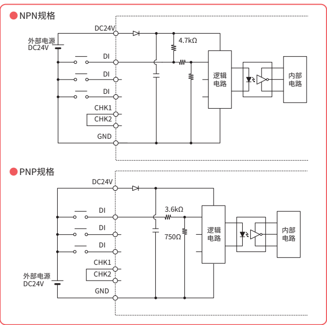
■ 输入信号连接示例
